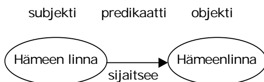
Kuva 3. RDF-lauseen osat
